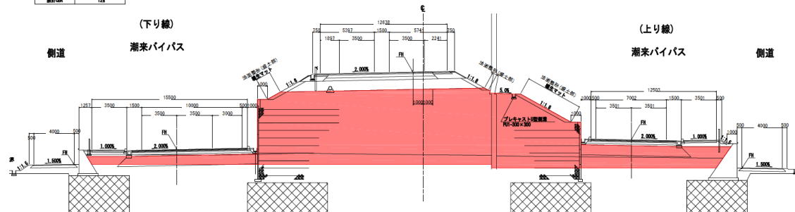
標準横断面図（交差点部） ※着色部：施工範囲
