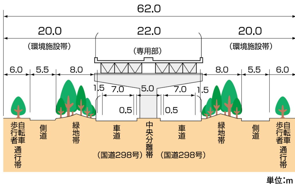
<標準断面>
